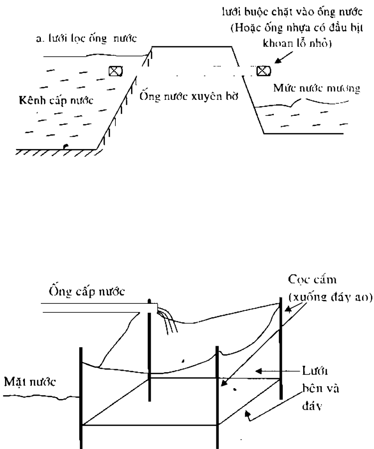
Hình 5b. – Bộ lọc cấp nước và lưới lọc cá tạp
