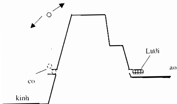
Hình 5b. – Bọng có cơ điều tiết nước
